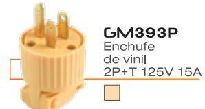
GM392S Toma de vinil 2P 125V 15A
